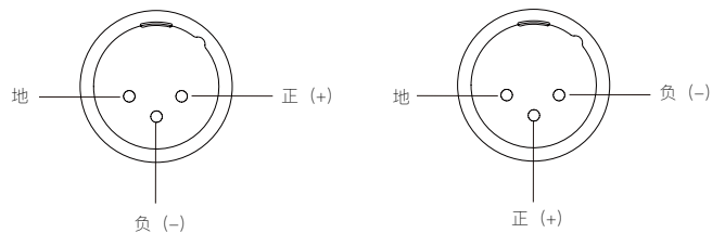
设置正向端口极性示意
