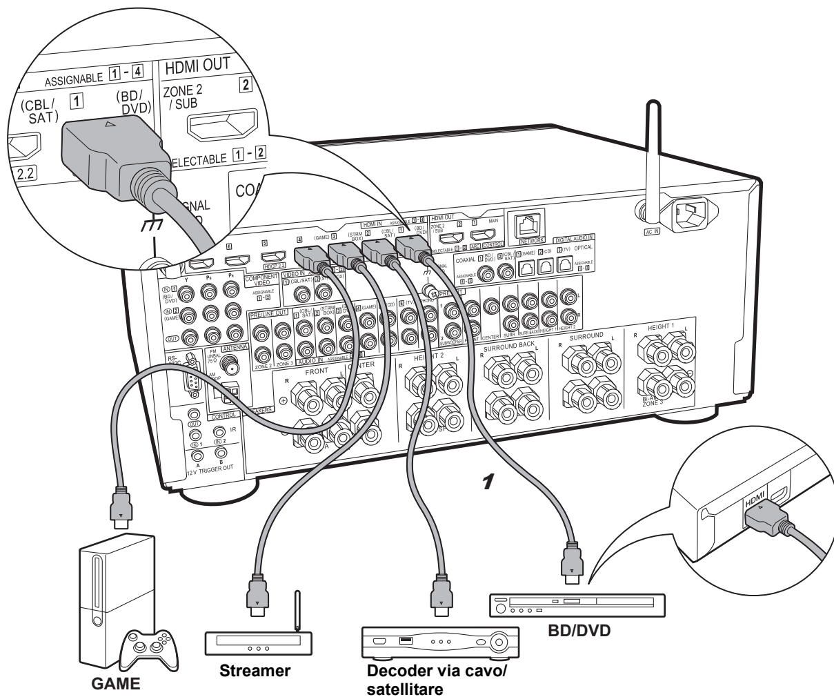
1 Cavo HDMI
