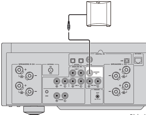
Rückseite
