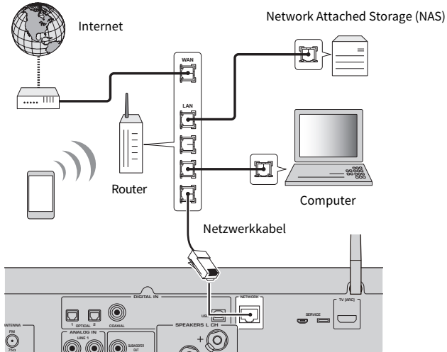
Rückseite
