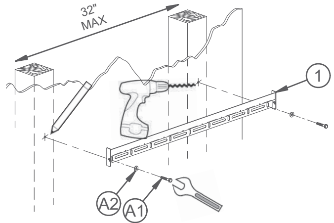
ii. Stud wall
